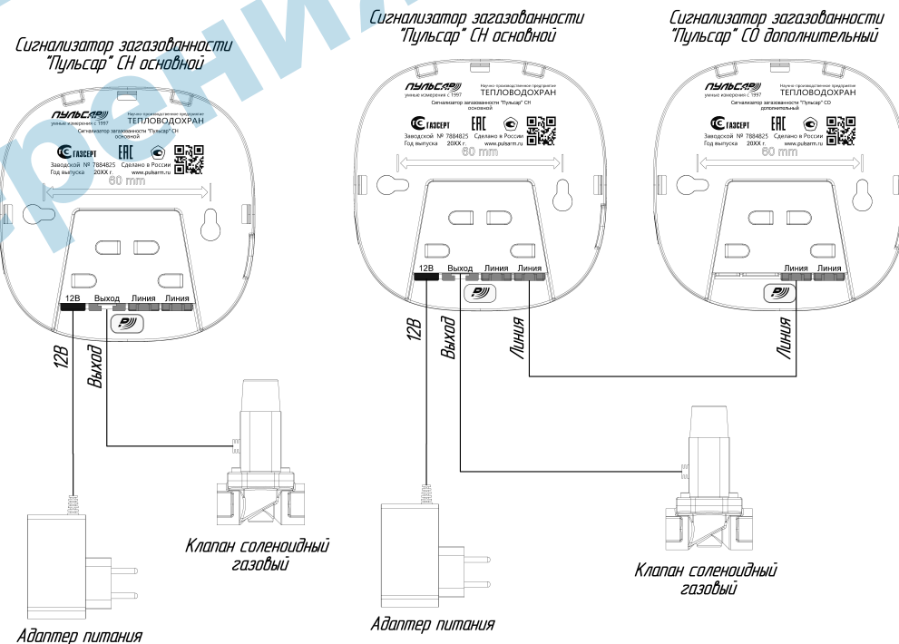
Рисунок 4 – Примеры конфигурации системы
