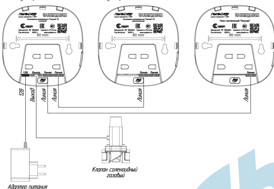
Сигнализатор загазованности "Пульсар" СН основной
