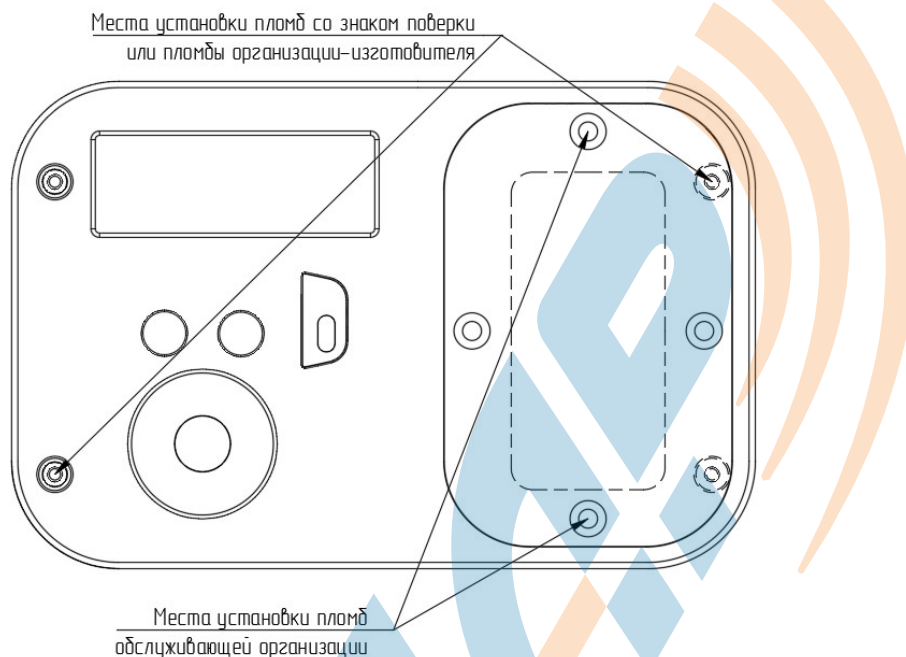
Рисунок 3 - Места установки пломб
