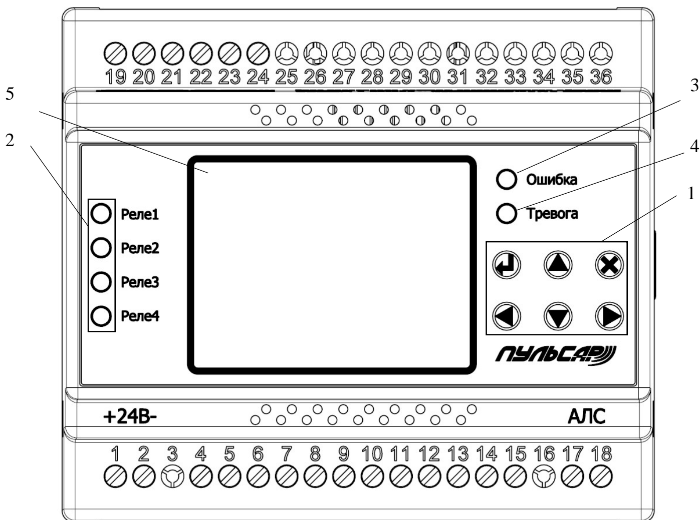
Рисунок 3 - Внешний вид блока управления системы сигнализаторов
