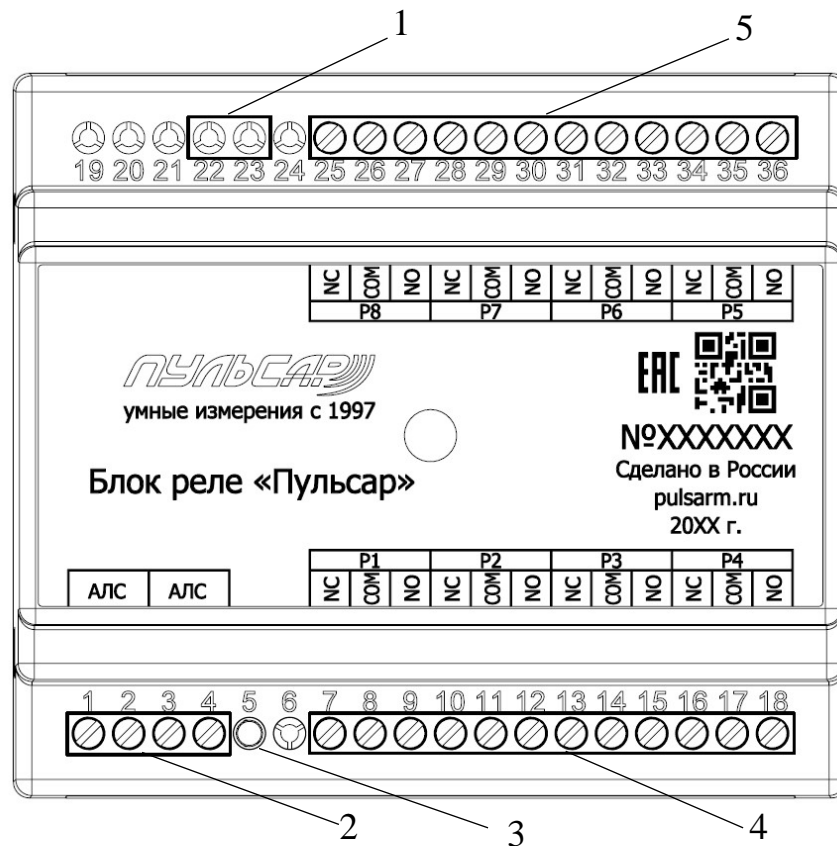
Рисунок 2 - Внешний вид блока реле
