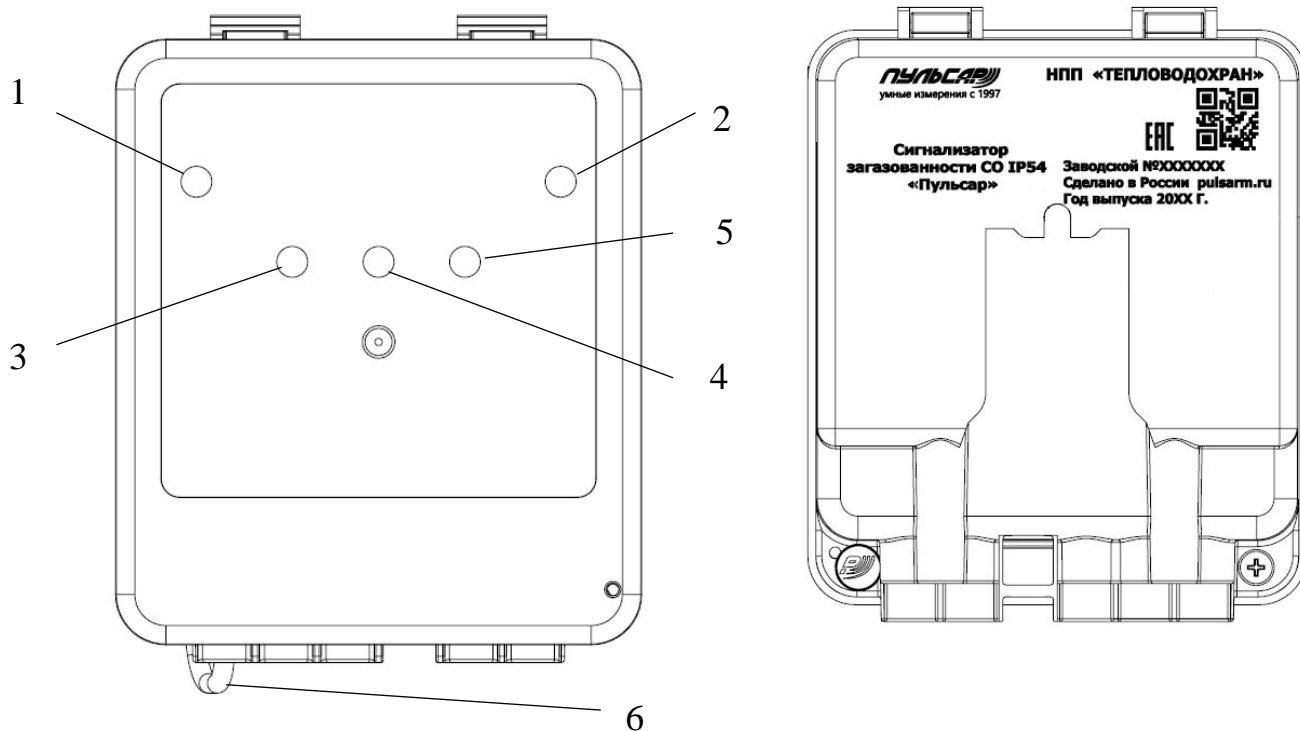
Рисунок 1 - Внешний вид сигнализатора ЮТЛИ.413415.051
