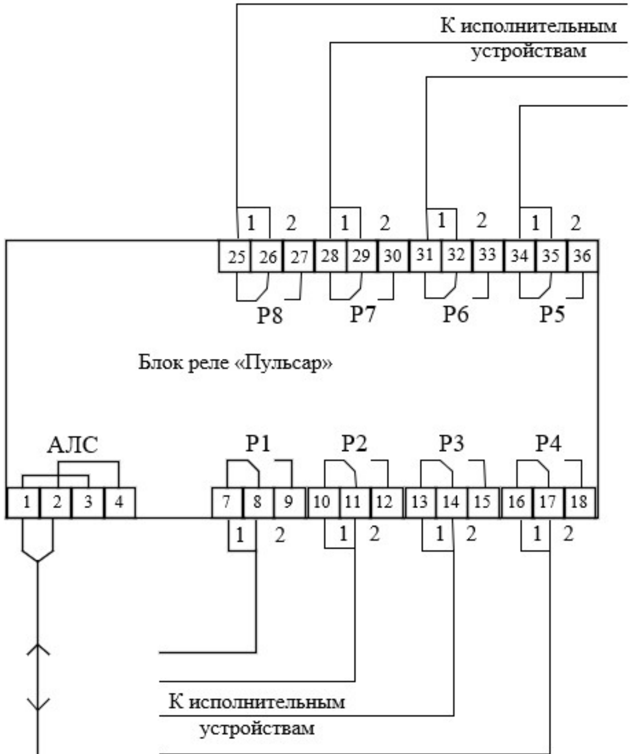
Схема подключения Блока реле «Пульсар»
