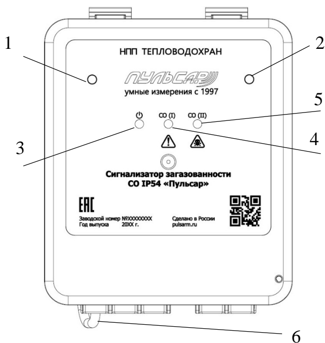
Рисунок 1в – Внешний вид сигнализатора ЮТЛИ.413415.049
