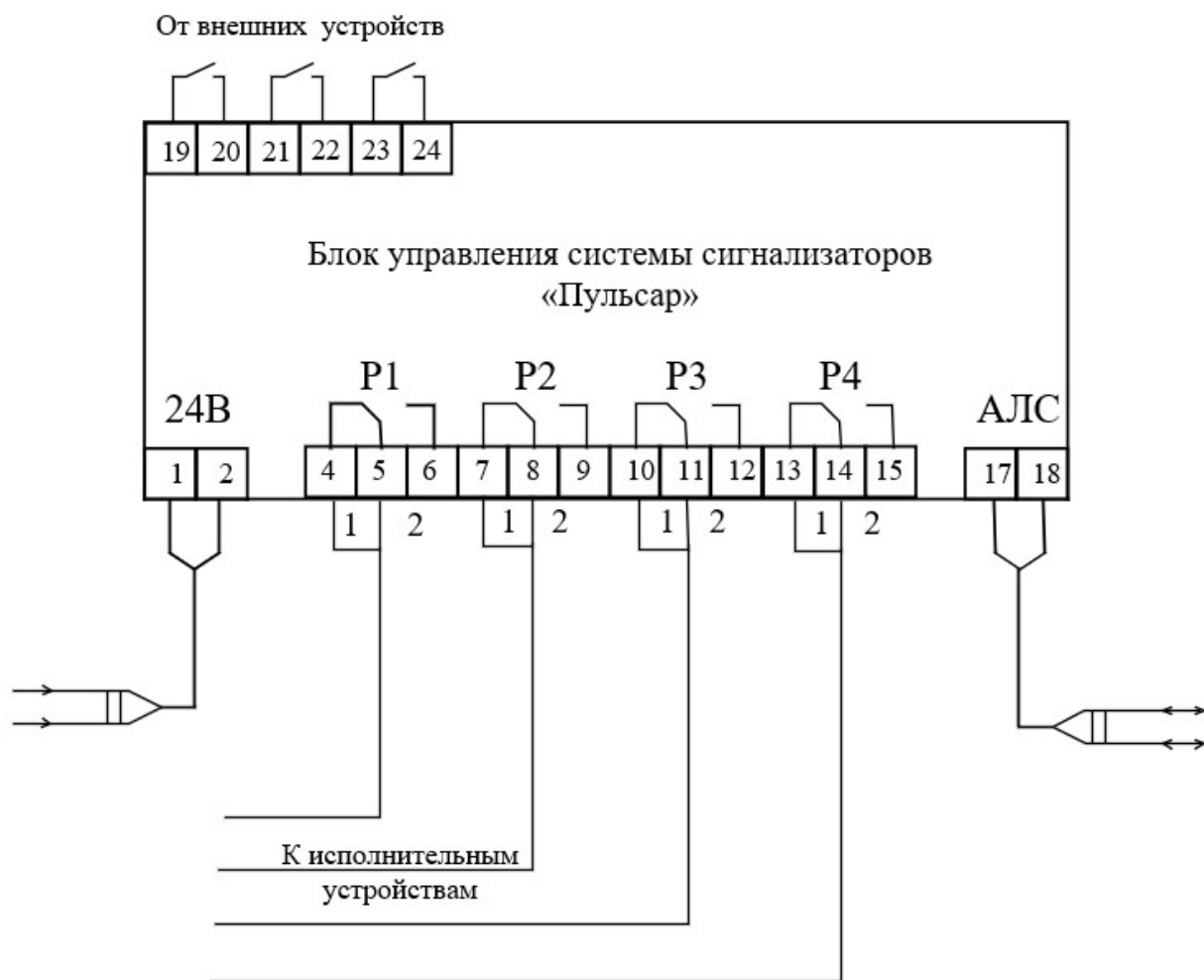
Схема подключения Блока управления системы сигнализаторов «Пульсар»
