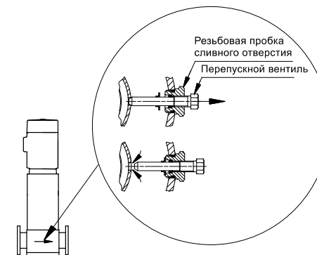
Рисунок 4 – Байпасный клапан
