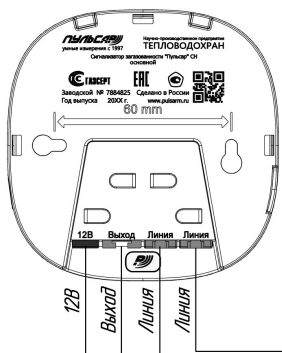
Сигнализатор загазованности "Пульсар" СН основной
