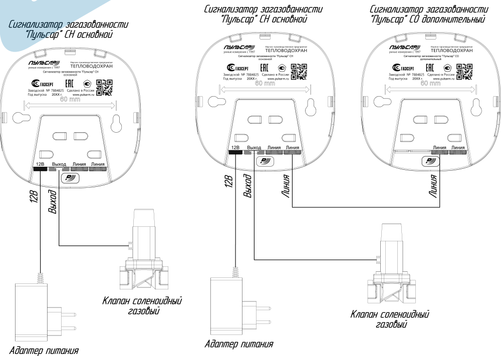
Рисунок 4 – Примеры конфигурации системы
