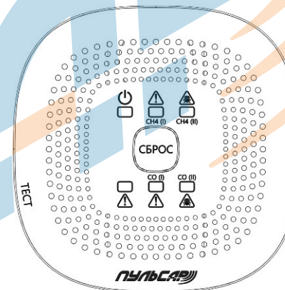
Рисунок 2 – Внешний вид пульта контрольного «Пульсар»
