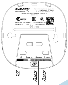
Сигнализатор загазованности "Пульсар" СН основной
