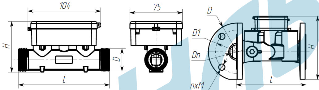
Приложение А ГАБАРИТНЫЙ ЧЕРТЕЖ И УСТАНОВОЧНЫЕ РАЗМЕРЫ
