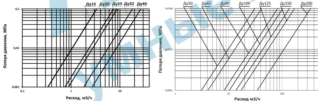
Приложение Б ДИАГРАММЫ ПОТЕРИ ДАВЛЕНИЯ
