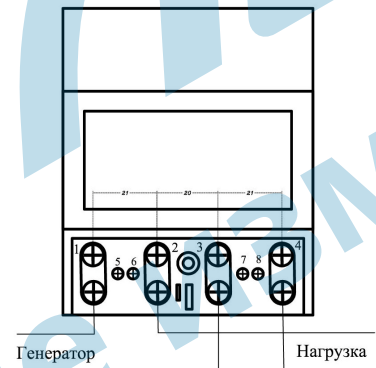
Приложение Б СХЕМА ВКЛЮЧЕНИЯ СЧЕТЧИКА
