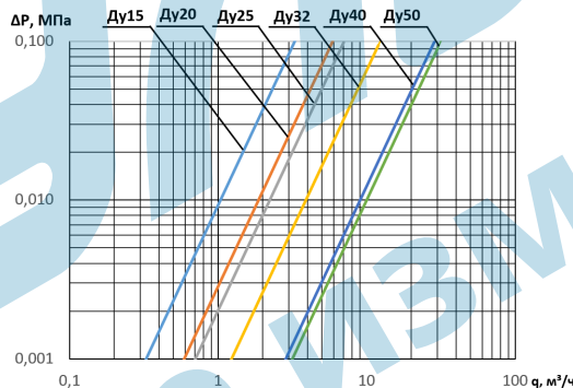
ПРИЛОЖЕНИЕ 2 Диаграмма потери давления
